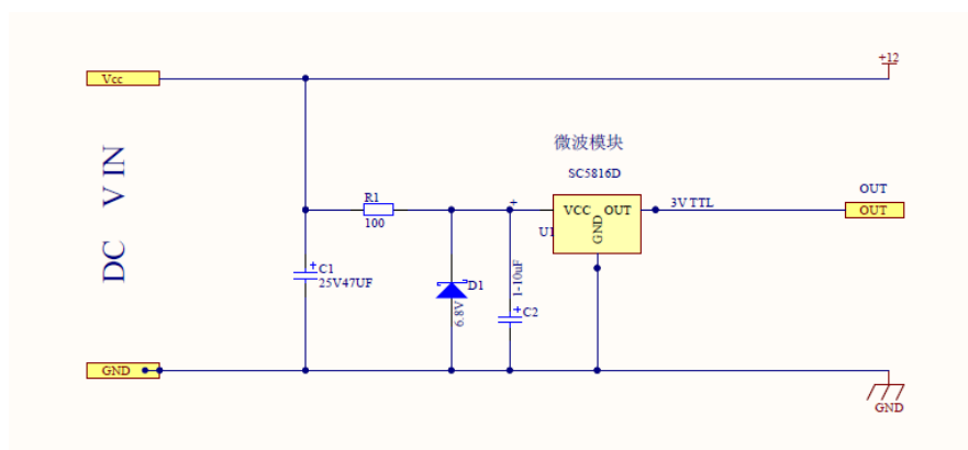
(微波雷达感应模块供电原理图)
